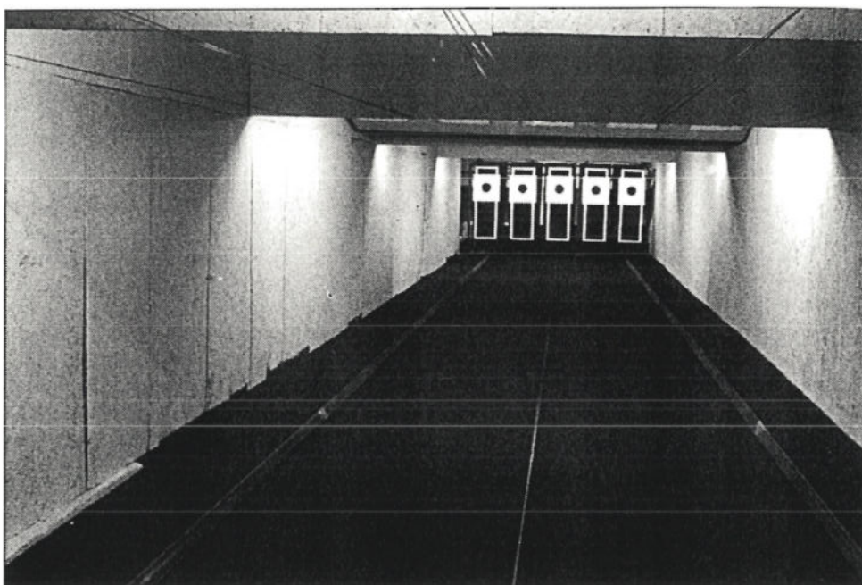
Der 25-m-Pistolenstand. Nach allen Erkenntnissen des Schießsportes erbaut.
